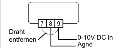
Abb. 8: Anschluss bei externem Stellsignal
