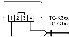
Schéma 4 : Raccordement des sondes de gaine et de sol en cas de fonctionnement avec une consigne interne
