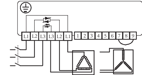
Abb. 1: Anschluss der Versorgungsspannung und Last
