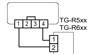
Figur 2: Inkoppling av rumsgivare TG-R5xx eller TG-R6xx vid drift med internt börvärde
