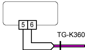
Abb. 7: Verdrahtung des Begrenzungsfühlers
