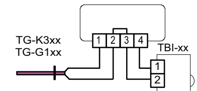
Schéma 6 : Raccordement en cas de sonde séparée externe et d'un potentiomètre TBI-xx comme réglage de consigne
