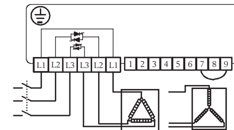
Abb. 1: Anschluss der Versorgungsspannung und Last
