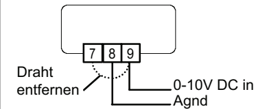
Abb. 8: Anschluss bei externem Stellsignal
