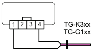
Abb. 4: Anschluss eines Fußboden oder Kanalfühlers bei Verwendung des internen Sollwertes.
