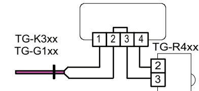
Schéma 5 : Raccordement en cas de sonde séparée externe et d'une TG-R4xx comme réglage de consigne seulement
