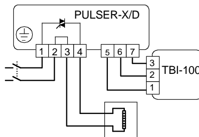
Figur 2 Manuellt inställbar modulering
