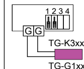
Figur 3 Omkopplarinställning och anslutning för internt börvärde och extern givare.
