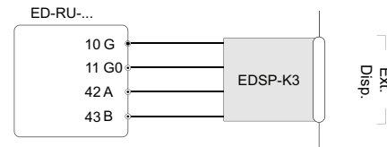
Bild 2 Verdrahtung mit einem EDSP-K3 Kabel
