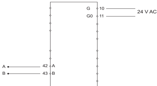
Bild 1 Verdrahtung
